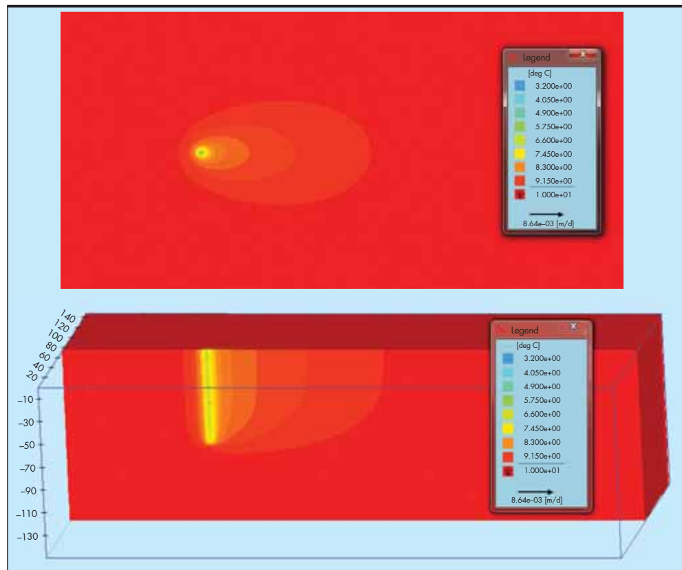
FIGURA 3. Temperatura del suelo de una sonda de extracción de 80 m en planta y en perfil, arena saturada con un flujo de 1 \cdot 10^{-7} m/s (0,0086 m/d) después de 20 años (en invierno).
