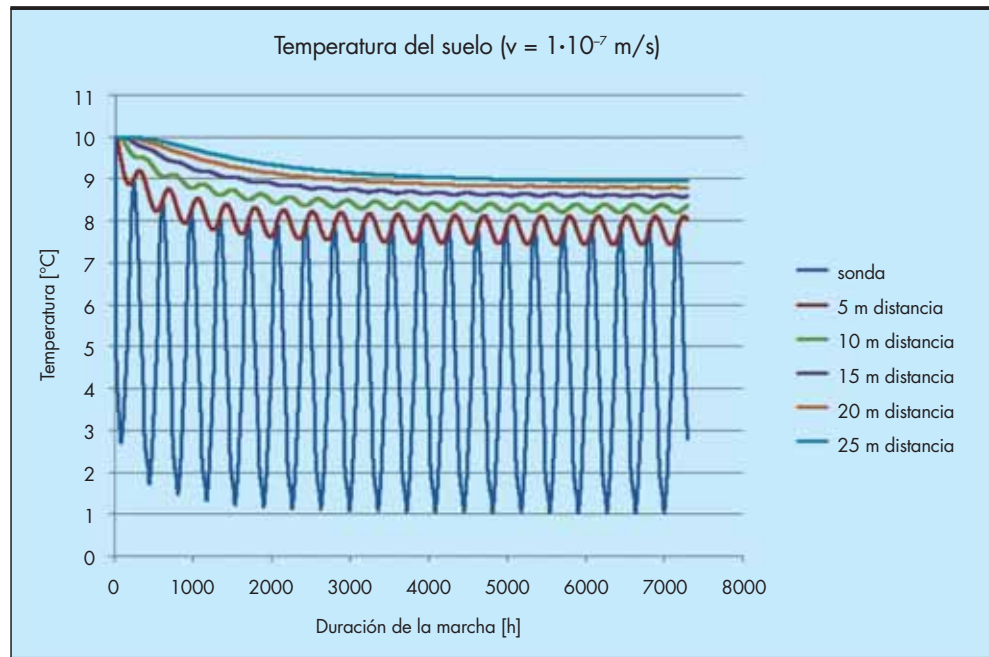
FIGURA 6. Temperatura del suelo en los puntos de observación de una sonda de extracción de 60 m, arena saturada con un flujo de 1 \cdot 10^{-7} m/s (0,0086 m/d).
