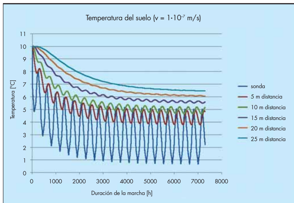
FIGURA 9. Temperatura del suelo en los puntos de observación de una planta de 5 sondas de sustracción de 95 m, arena saturada con una corriente de 1 \cdot 10^{-7} m/s ( 0,086 m/d), relativamente a la sonda del medio.
