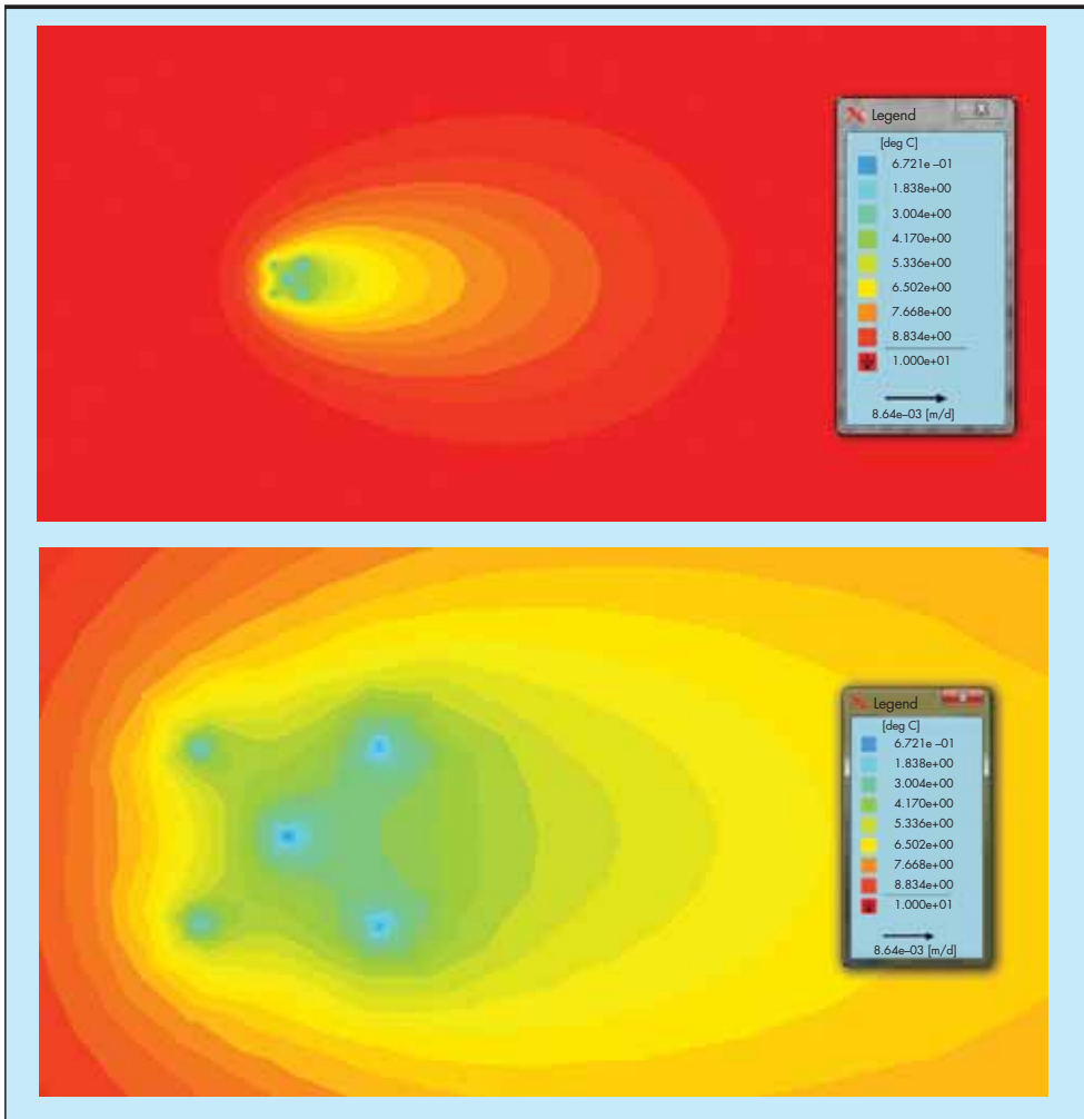
FIGURA 8. Temperatura del suelo de una instalación de 5 sondas de extracción de 95 m, arena saturada con una corriente de 1 \cdot 10^{-7} m/s ( 0,0086 m/d) después de 20 años (en invierno).
