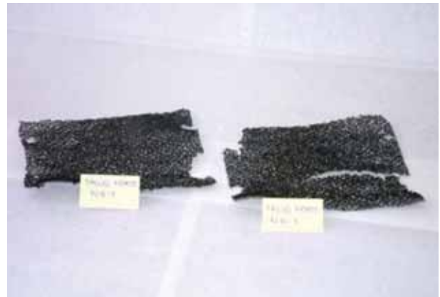
FIGURA 11. Estado de las probetas extraídas de obra tras el ensayo en medio alcalino.
