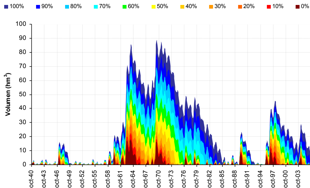
Figura 10. Escenarios simulados de reducción de aportes subterráneos a la laguna de Fuente de Piedra. Fuente: INTECSA-INARSA.
