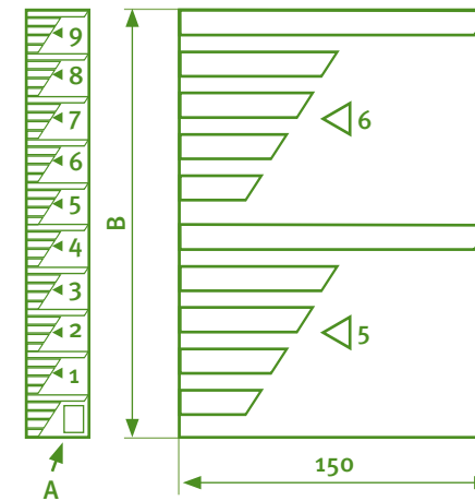
Figura a1. Detalle de la escala graduada de una escala limnimétrica. Detalle de la placa desmontable para las cifras de la graduación de color rojo (A) y divisiones de 10 mm (B).
